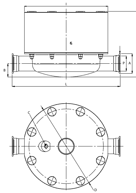
Amortisseur en Acier inox, version sanitaire
